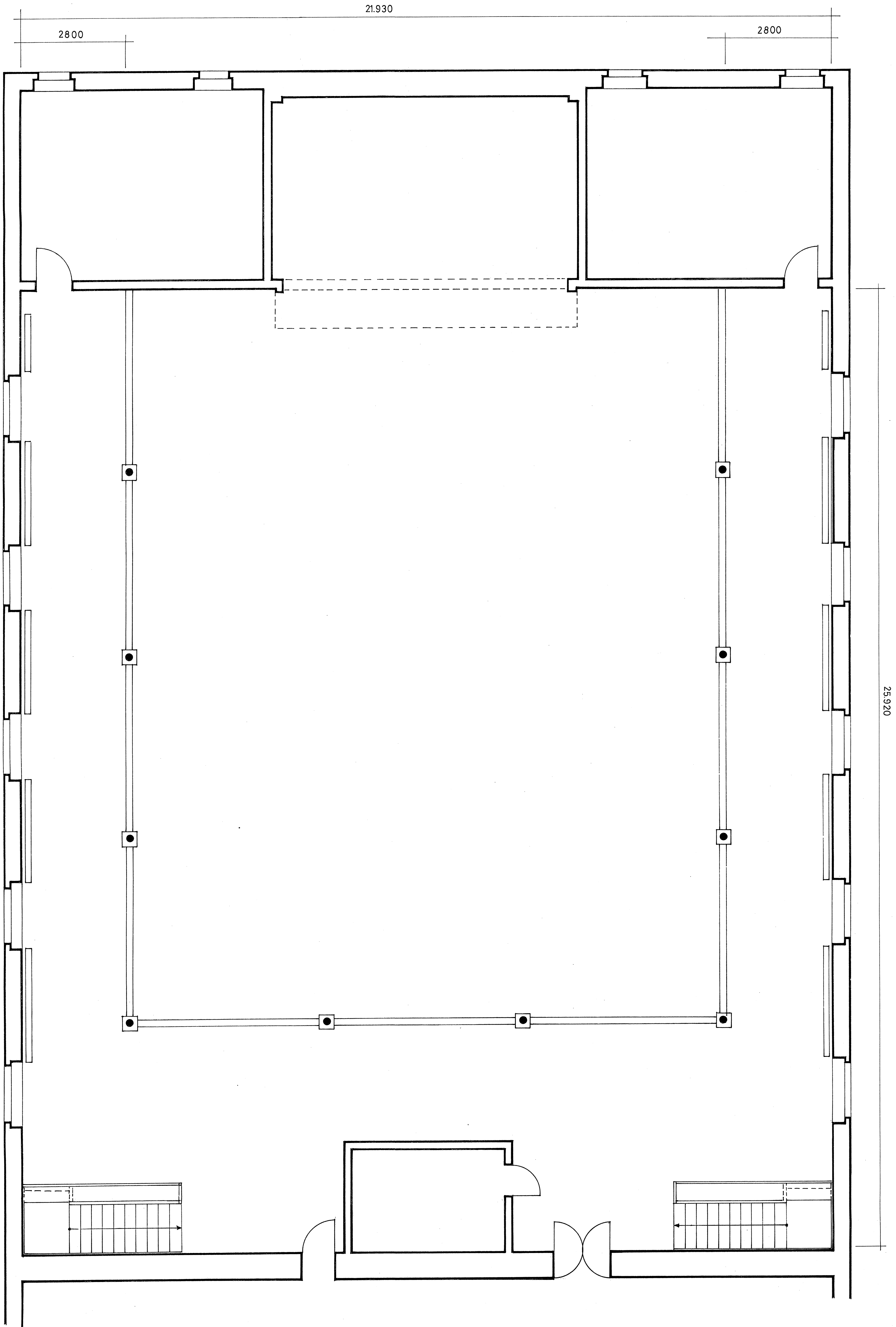
GRUNDRISS GROSSER SAAL GALERIE
