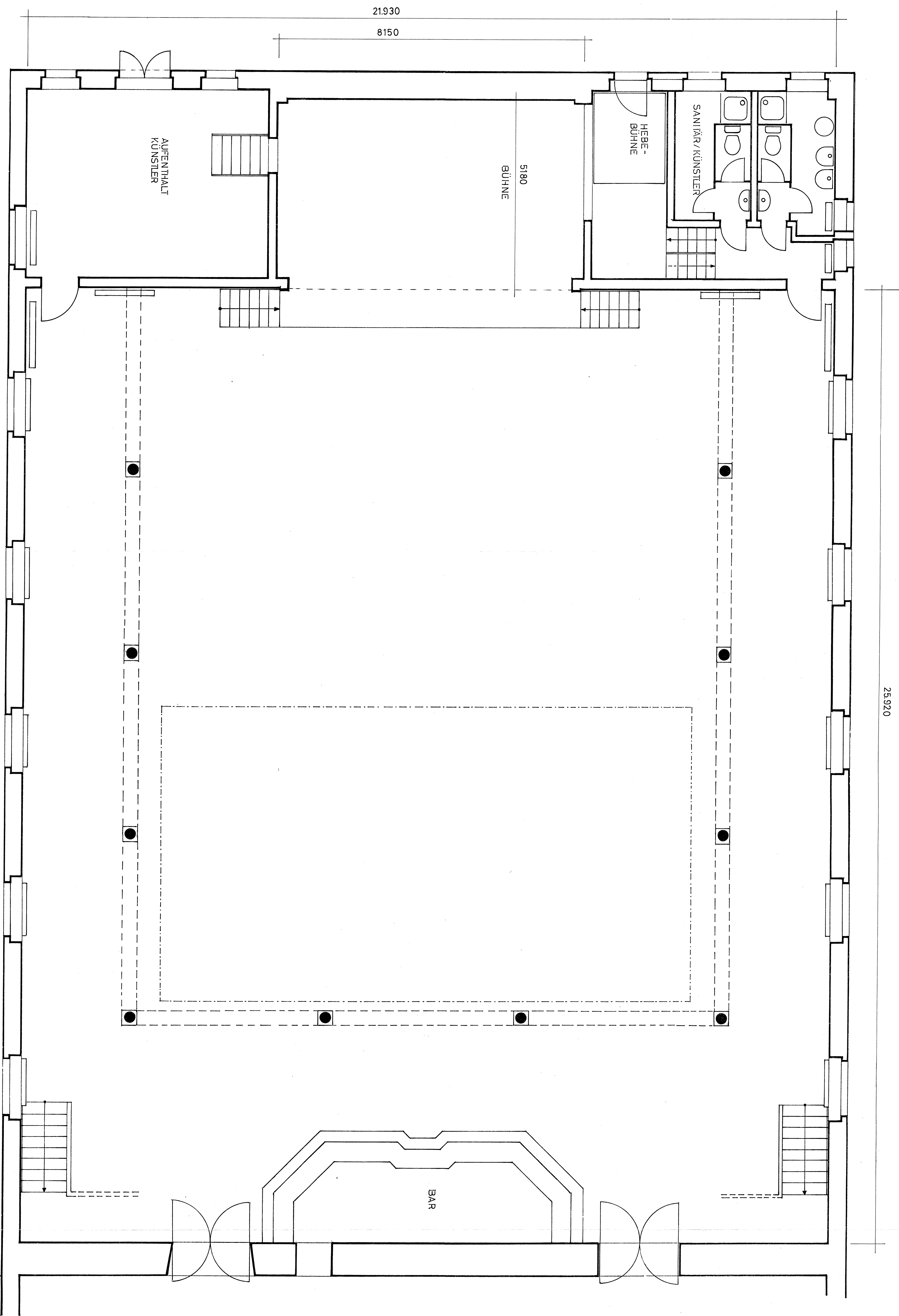
GRUNDRISSE GROSSER SAAL M.1:50
